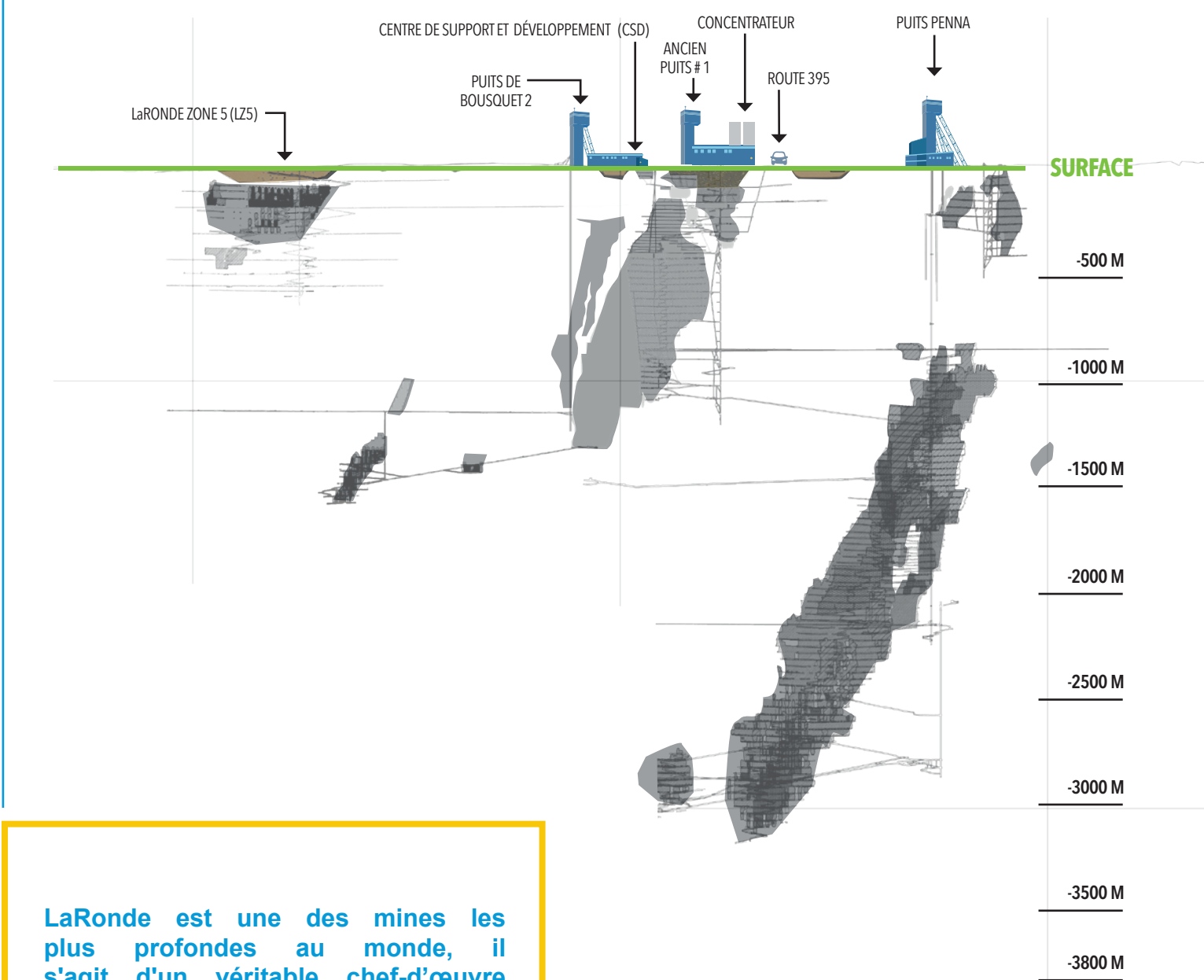
FIGURE 2 : VUE LONGITUDINALE DES GISEMENTS DU COMPLEXE MINIER LaRONDE
